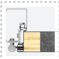
Ościeżnica PERFOTHERM 50*
