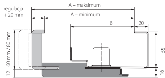
przekrój ościeżnicy PROJEKT Premium
